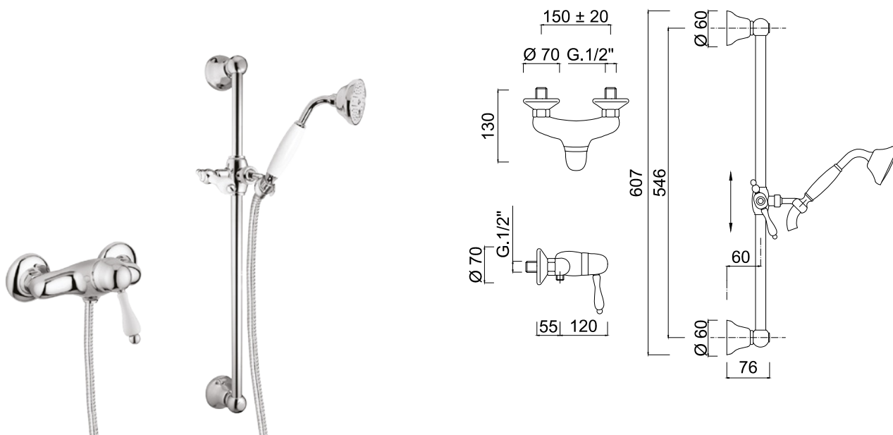
Cartuccia ceramica Ceramic cartridge
