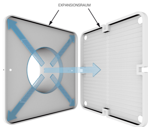
LUFTSTROM BEI AirDecor LÜFTUNGSGITTERN
